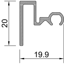
Profil No : D1-505 ⚠ Ağırlık : 199 gr/m ⚠ İşaretili profil için satış ekibinden bilgi alınır.
