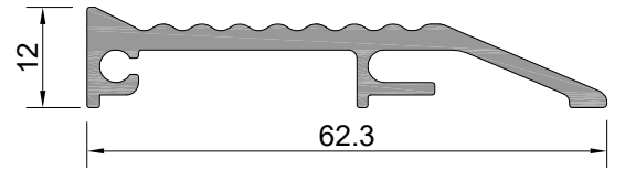
Profil No: W-545 Ağırlık : 578 gr/m
