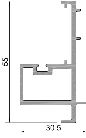
Profil No : W4-506 ⚠ Ağırlık : 698 gr/m ⚠ İşaretili profil için satış ekibinden bilgi alınız.
