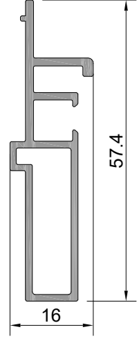
Profil No : W3-511 ⚠ Ağırlık : 496 gr/m ⚠ İşaretili profil için satış ekibinden bilgi alınız.
