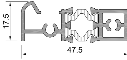
Profil No : W-555 Ağırlık PVC : 767 gr/m Ağırlık POLY : 758 gr/m
