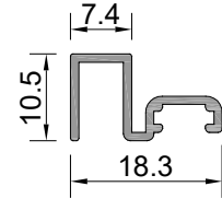
Profil No : W-556 ⚠ Ağırlık : 126 gr/m ⚠ İşaretili profil için satış ekibinden bilgi alınır.
