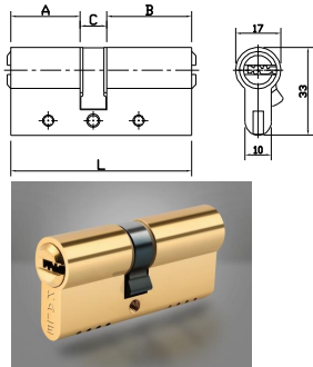
D-851 (yerli) naturel D-852 (yerli) pres-renkli boyalı
