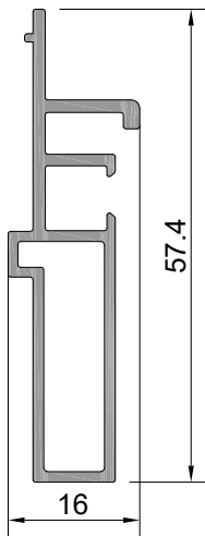
Profil No : W3-511 ⚠ Ağırlık : 496 gr/m ⚠ İşaretti profil için satış temsilcinizden bilgi alınız.
