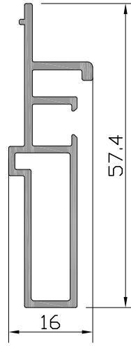
Profil No: W-558 Ağırlık : 173 gr/m
